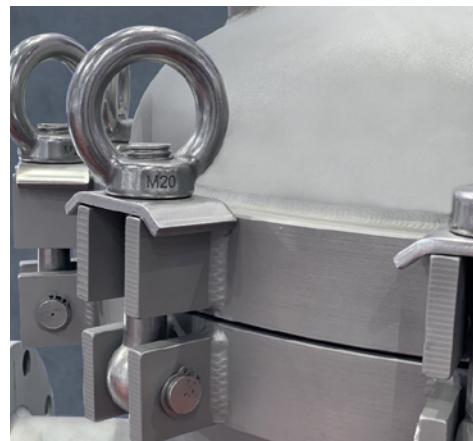
标准多袋式过滤器产品细节图
